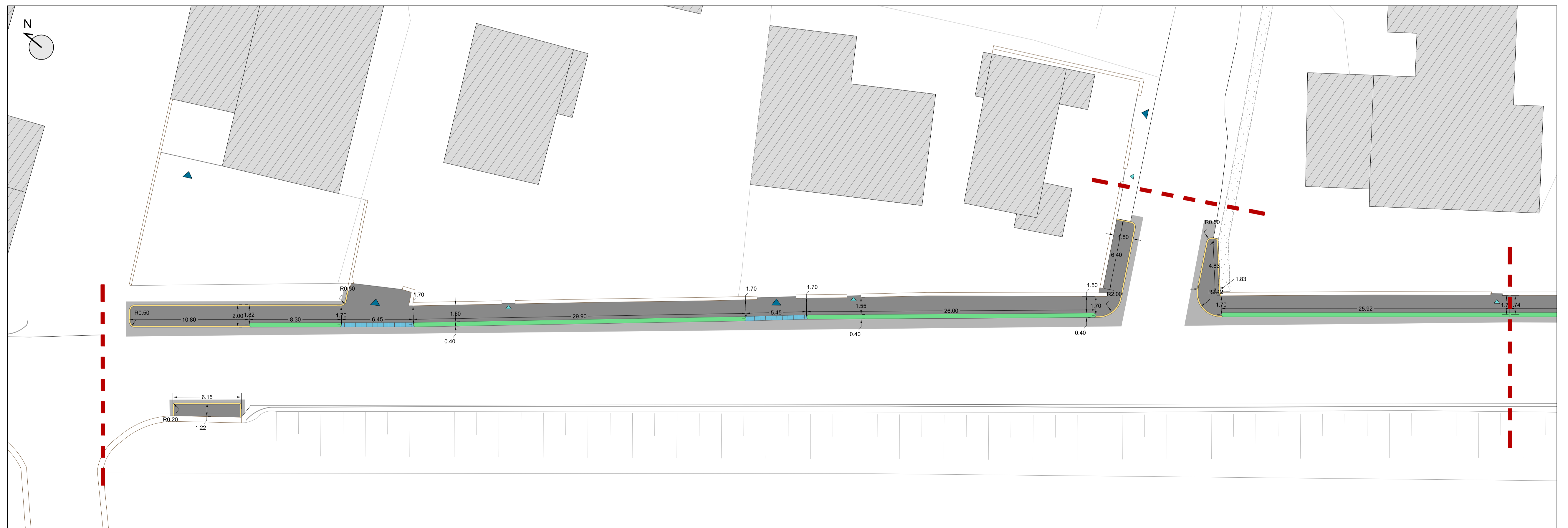
Planimetria 02 - Tracciamenti e asfaltature, scala 1:200
