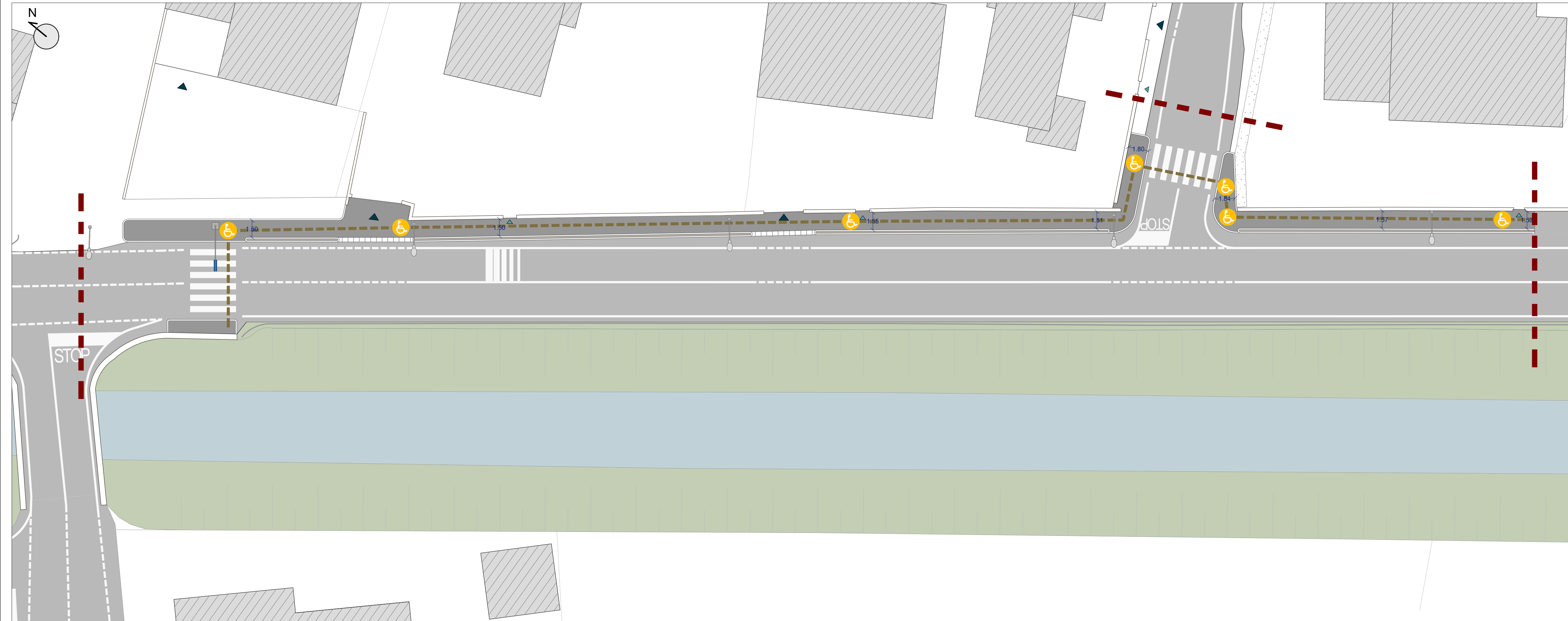
Planimetria - scala 1:200
