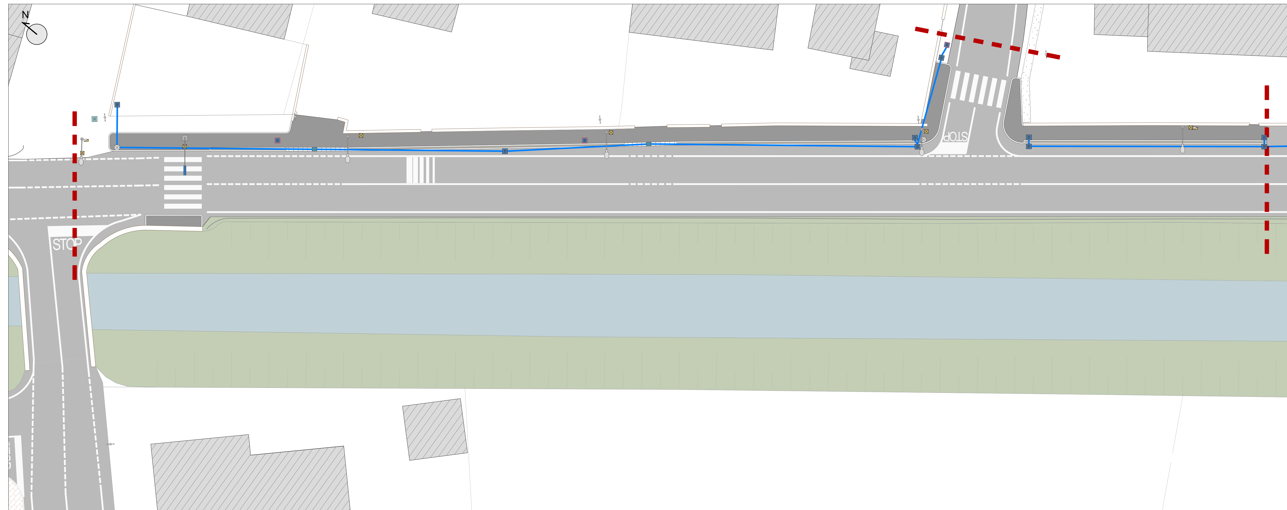
Planimetria schema rete acque bianche - scala 1:200
