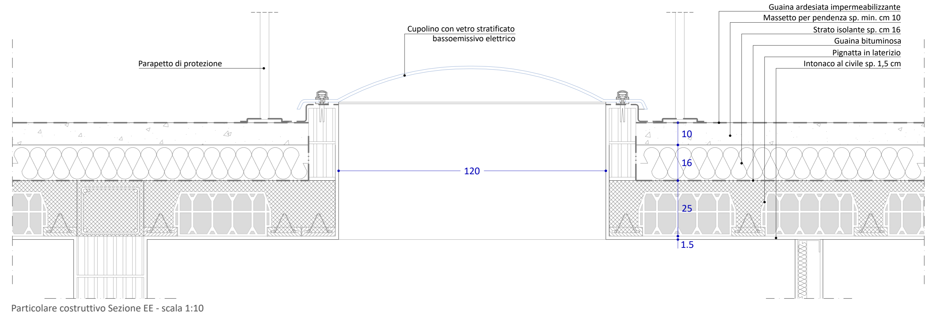
Particolare costruttivo Sezione EE - scala 1:10
