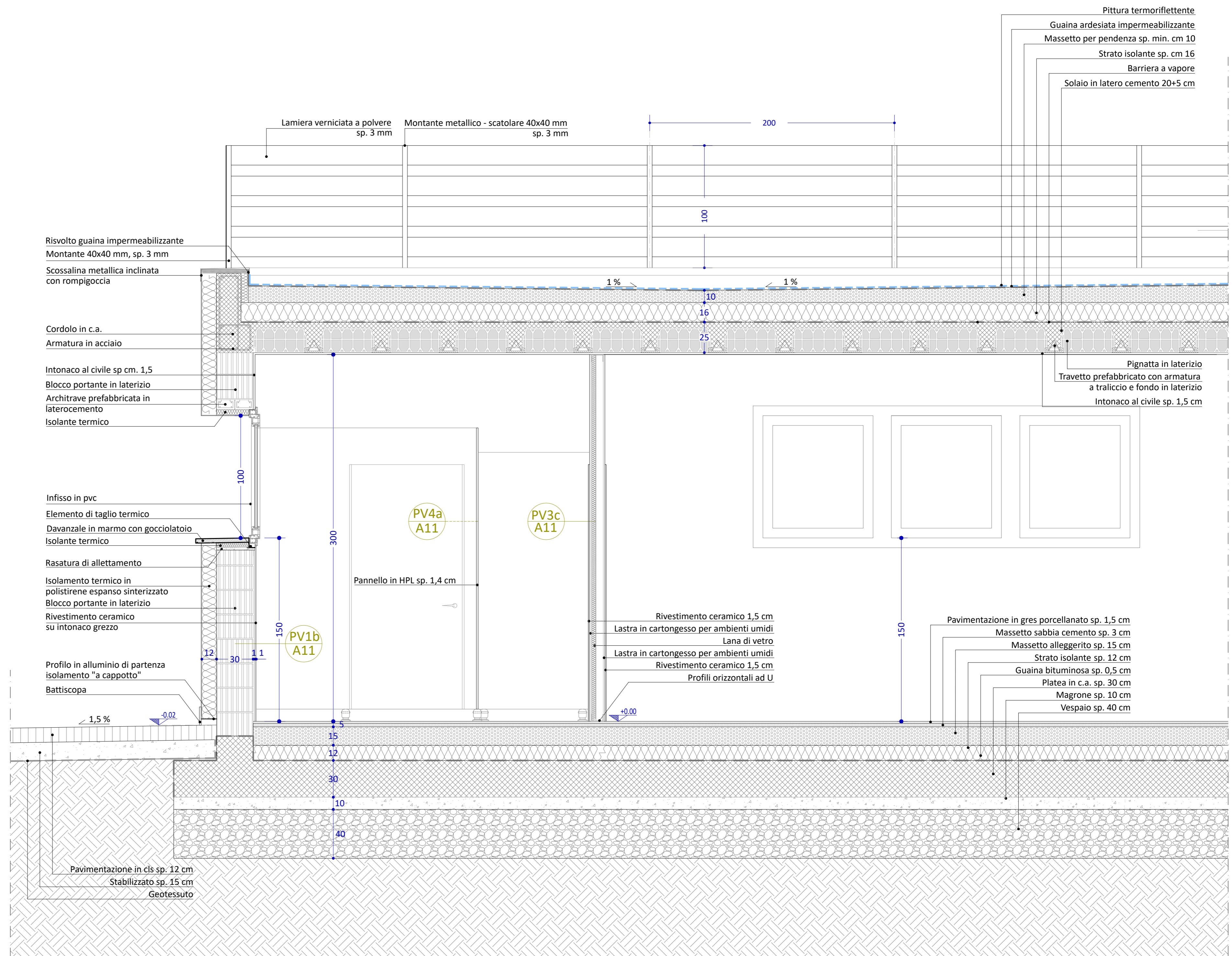
Particolare costruttivo Sezione AA - scala 1:20
